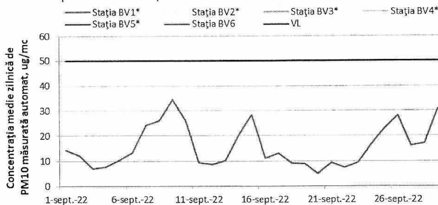
Figura 1.1.2.4.1. Evoluția mediilor zilnice de PM 10, metoda automată, în luna septembrie
