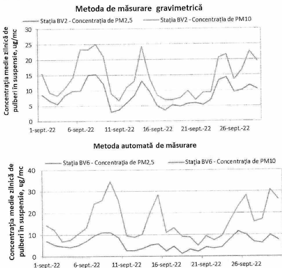
Figura 1.1.2.4.4 Evoluția mediilor zilnice de PM 2,5 și PM10 în luna septembrie
