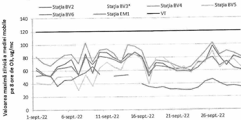
Figura 1.1.2.3.1. Evoluția maximelor zilnice ale mediilor mobile pe 8 ore de \text{O}_3 în luna septembrie
