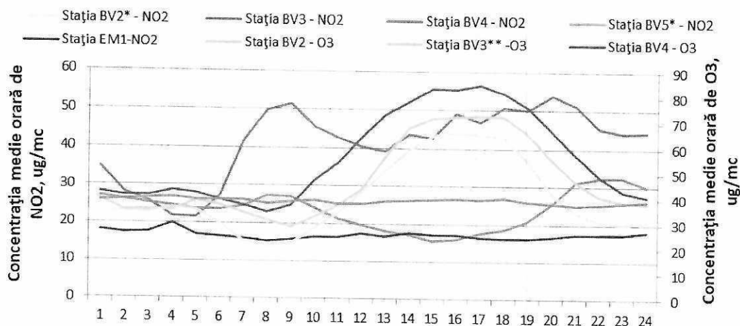
Figura 1.1.2.3.3. Ciclul zilnic al O 3 și NO 2
