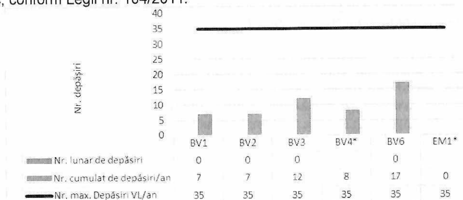
Figura 1.1.2.4.2 Numărul lunar și cumulat de depășiri ale valorii limită zilnice la PM10
