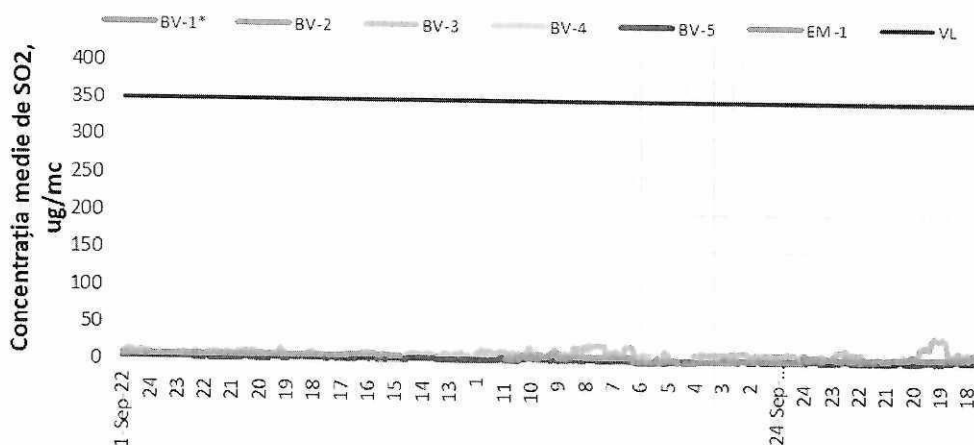
Figura 1.1.2.1.2. Evoluția mediilor orare de SO 2 în luna septembrie
