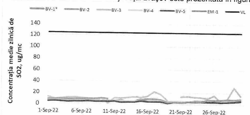
Figura 1.1.2.1.1. Evoluția mediilor zilnice de SO 2 în luna septembrie
