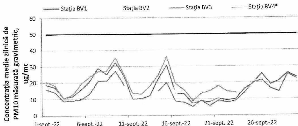
Figura 1.1.2.4.1. Evoluția mediilor zilnice de PM 10 (gravimetric) în luna septembrie
